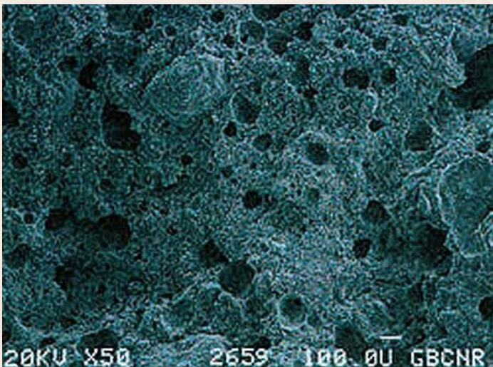
Snímka základného vrstvy Rinzaffo MGN zo skenovacieho elektrónového mikroskopu ukazuje svoju jedinečnú mikropórovú štruktúru
